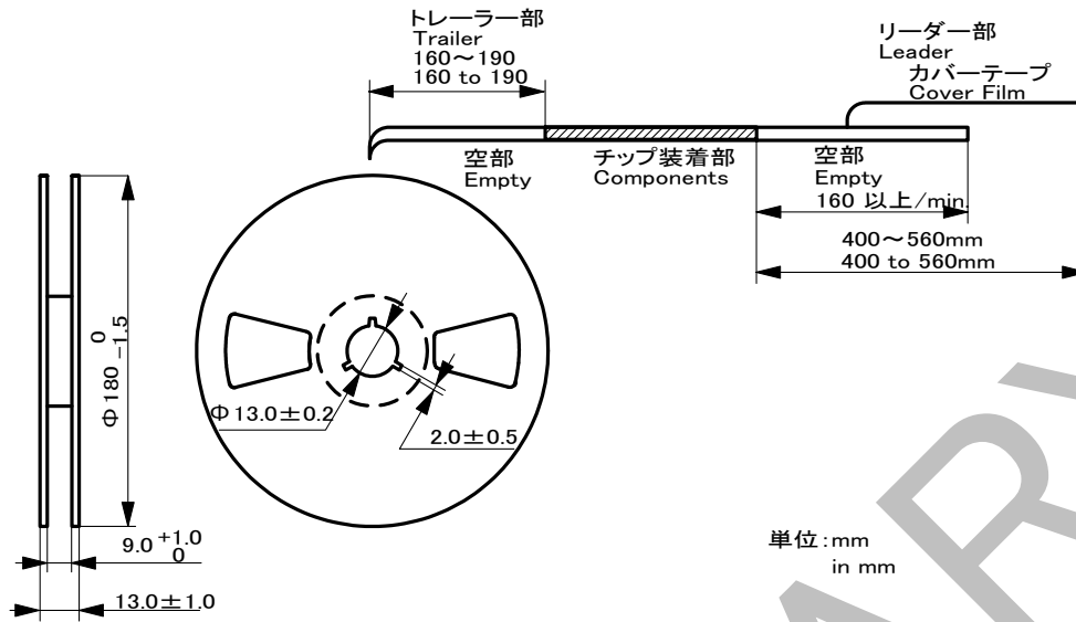
第6図 プラスチックリールの外形寸法図 Figure 6. Dimensions of Plastic Reel
