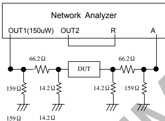
第1-1図 周波数測定回路 Figure 1-1 Frequency measuring circuit
