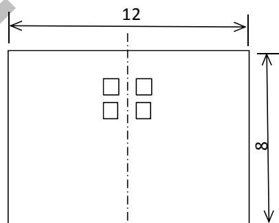
第3図 たわみ試験用プリント基板 Figure 3. PCB for Bending Strength Test
