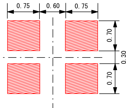
第2図 外形寸法図
